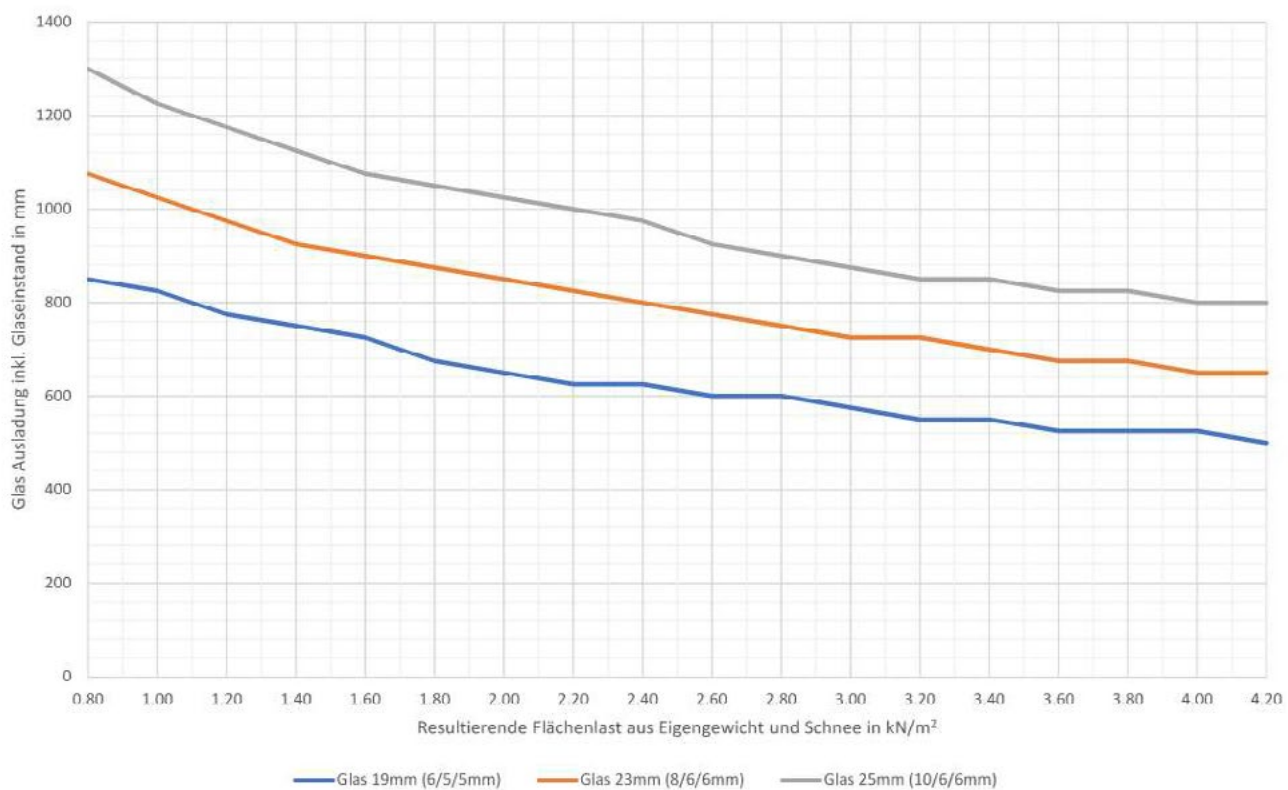
Glasdiagramm zu Bezugshöhe 600 Meter
