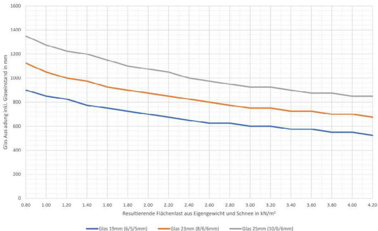
Glasdiagramm zu Bezugshöhe 500 Meter
