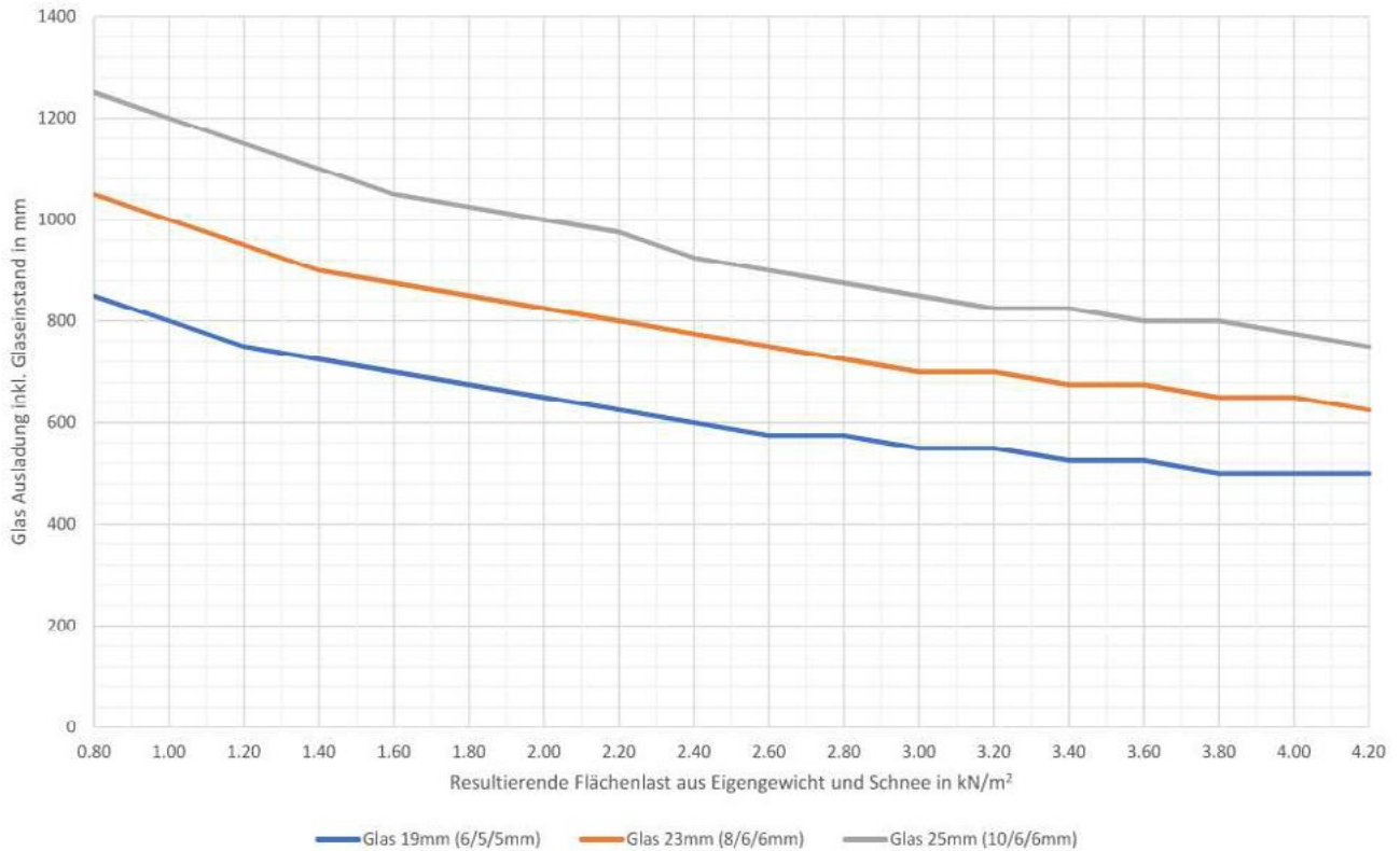
Glasdiagramm zu Bezugshöhe 700 Meter
