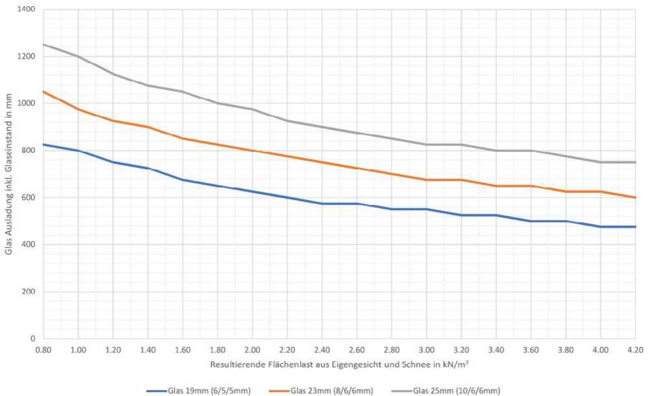
Glasdiagramm zu Bezugshöhe 800 Meter
