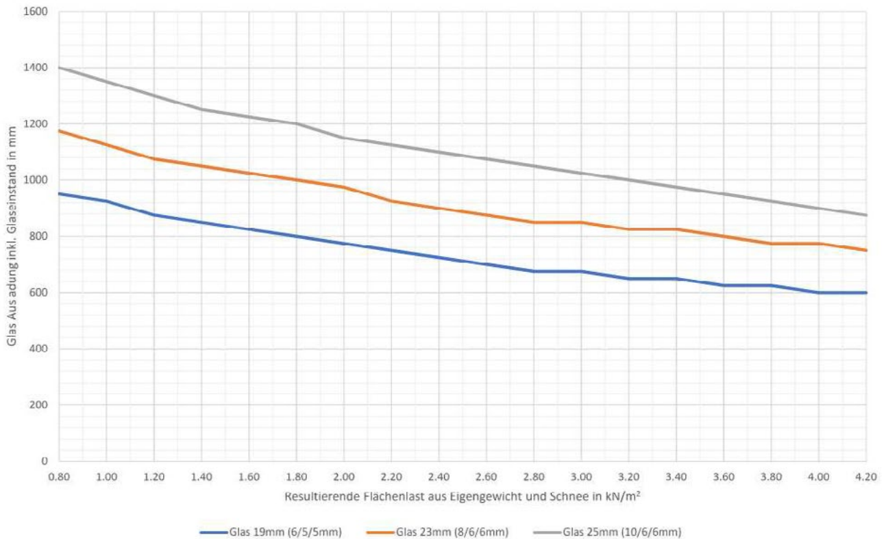
Glasdiagramm zu Bezugshöhe 400 Meter
