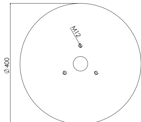
Anschlussplatte mit aufgeschweisstem Aussengewinde, Dicke 8 mm
